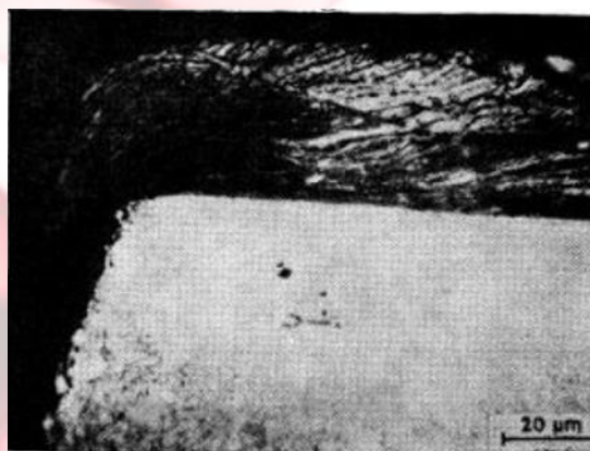
Рис. 1 – Сечение по наросту на твердосплавном инструменте после обработки резанием серого чугуна с пластинчатым графитом.
